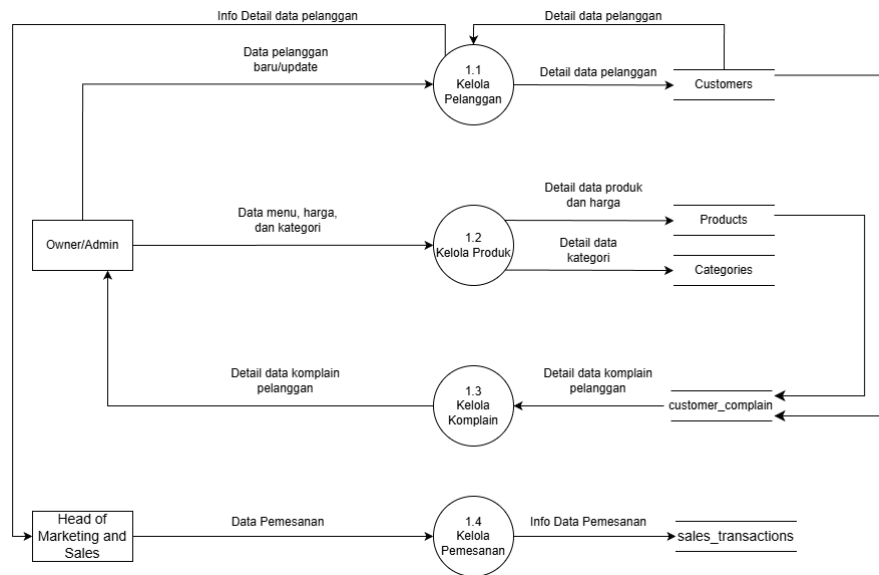
Gambar 66. DFD Level 2.1 (Penjualan)
