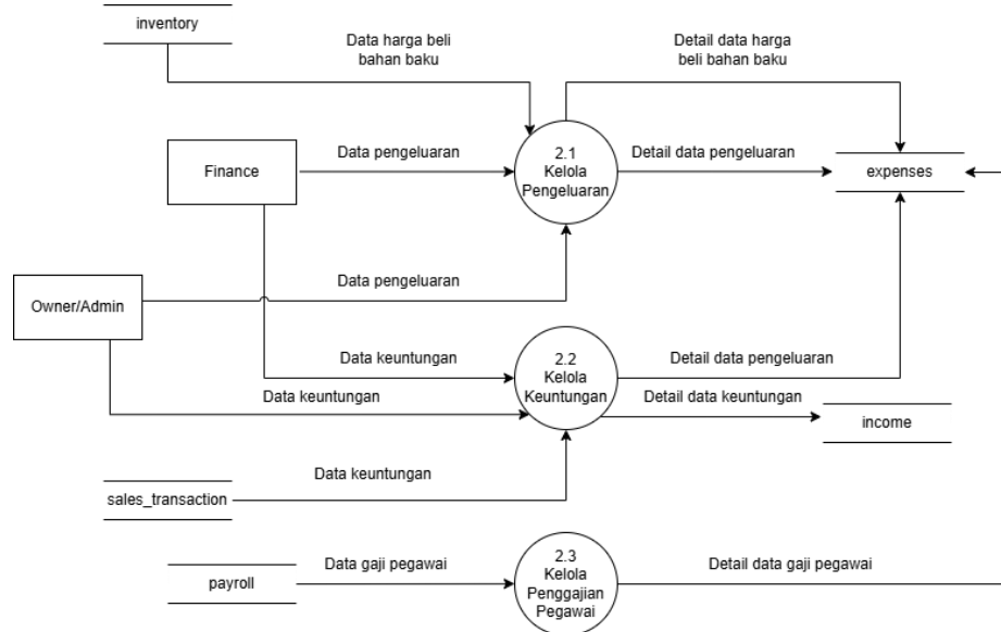
Gambar 77. DFD Level 2.2 (Proses Keuangan dan Akuntansi)
