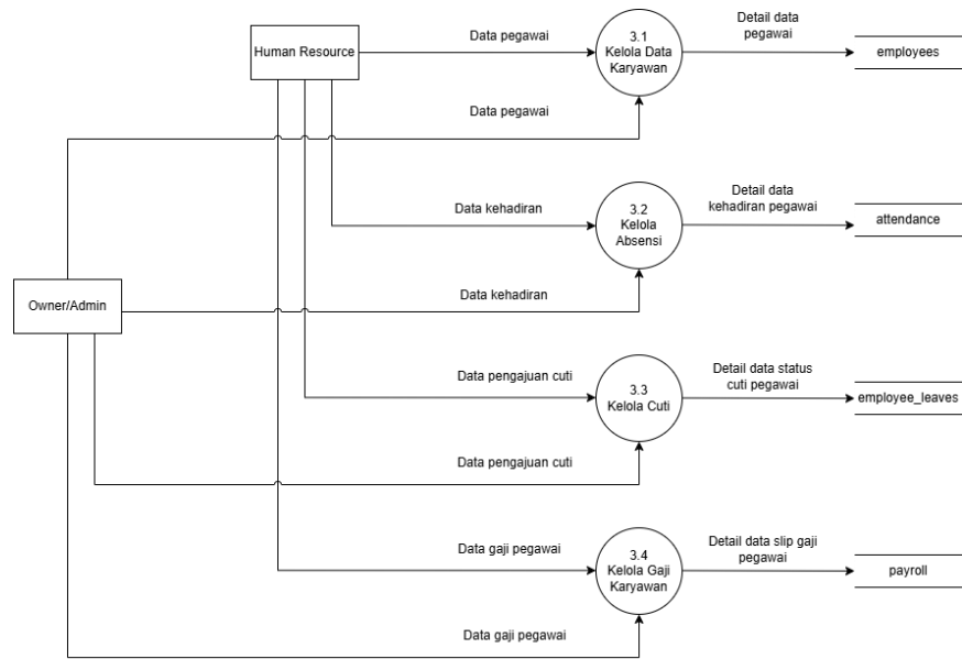
Gambar 88. DFD Level 2.3 (Pengelolaan Pegawai)
