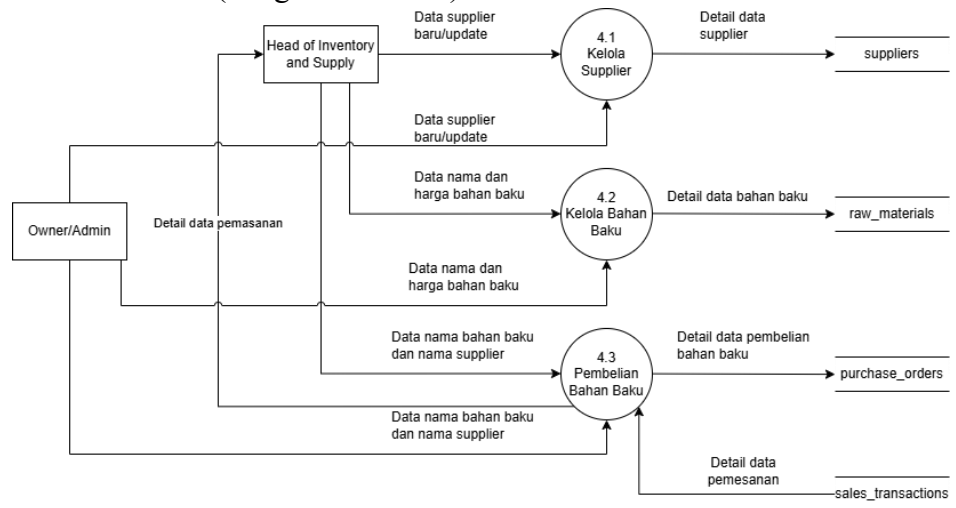
Gambar 99. DFD Level 2.4 (Pengelolaan Stok)
